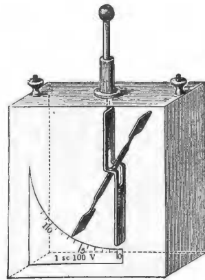
Fig. 1353a, Nos. 33315/19.
